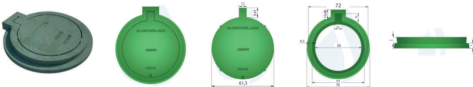
Aro Tapa pozo peatonal
