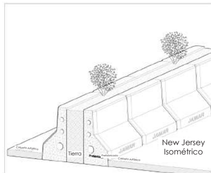
Barrera Monodireccional New Jersey
