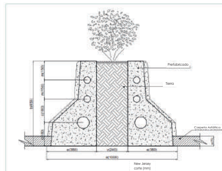
Barrera Monodireccional New Jersey
